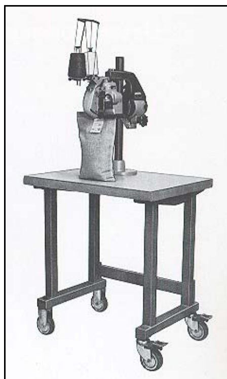
Klasse 2200AT mit Pedestal H1400T und Stahlprofil Tisch A9847B
