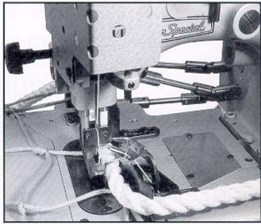
81500CZ3374B FÜR 10-16 mm SEILE
