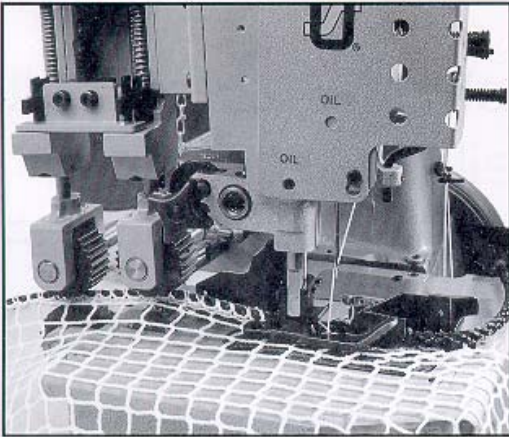
81500CZ3374A FÜR 4 - 12 mm SEILE
