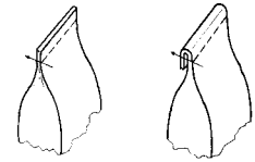
Umschlag-Verschluss von Hand durch Bediener oder durch zusätzliche Sackzuführeinrichtung mit Sackumfalteinrichtung
